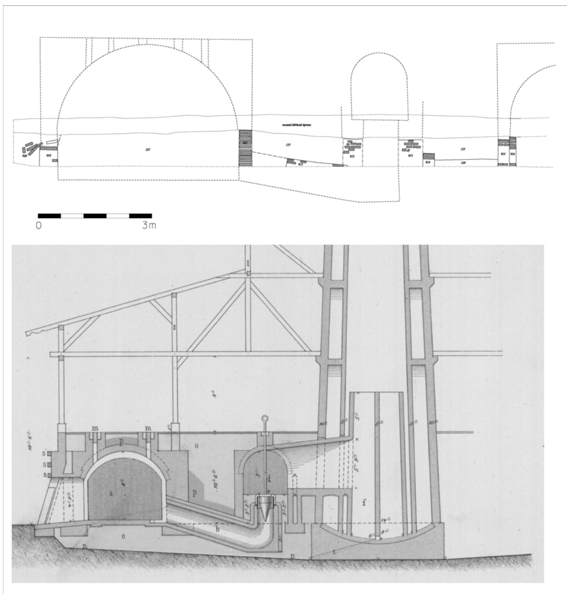
Obr. 7 Nahore částečně rekonstruovaný řez západní částí pece s vypalovací komorou, odtahovým kanálem a předpokládaným kouřovým sběračem. Dole řez kruhovou pecí podle Loeffa 1870
