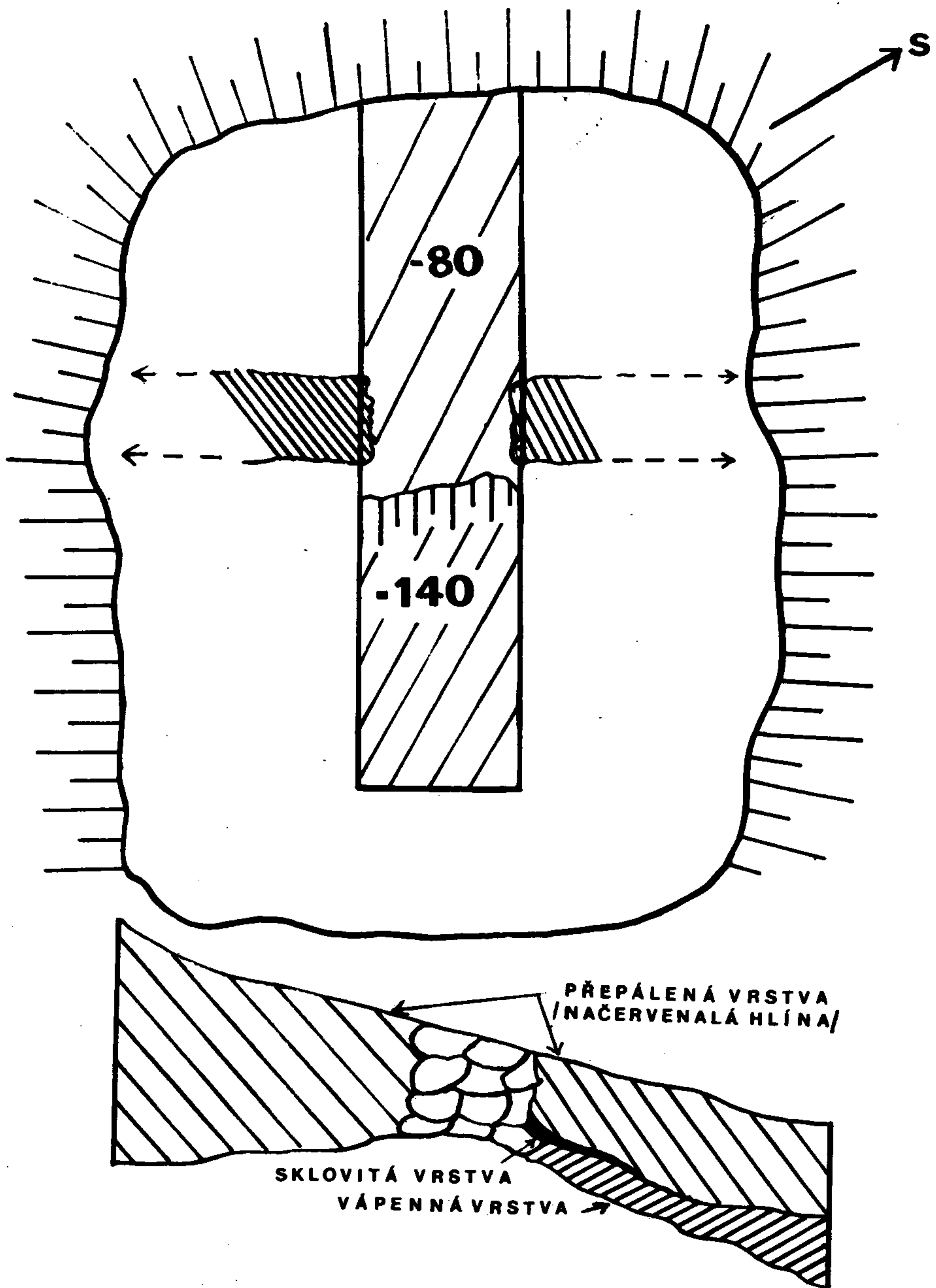
Půdorys a řez středověké vápenické pece u hradu Šaumberku (kresba autor)
